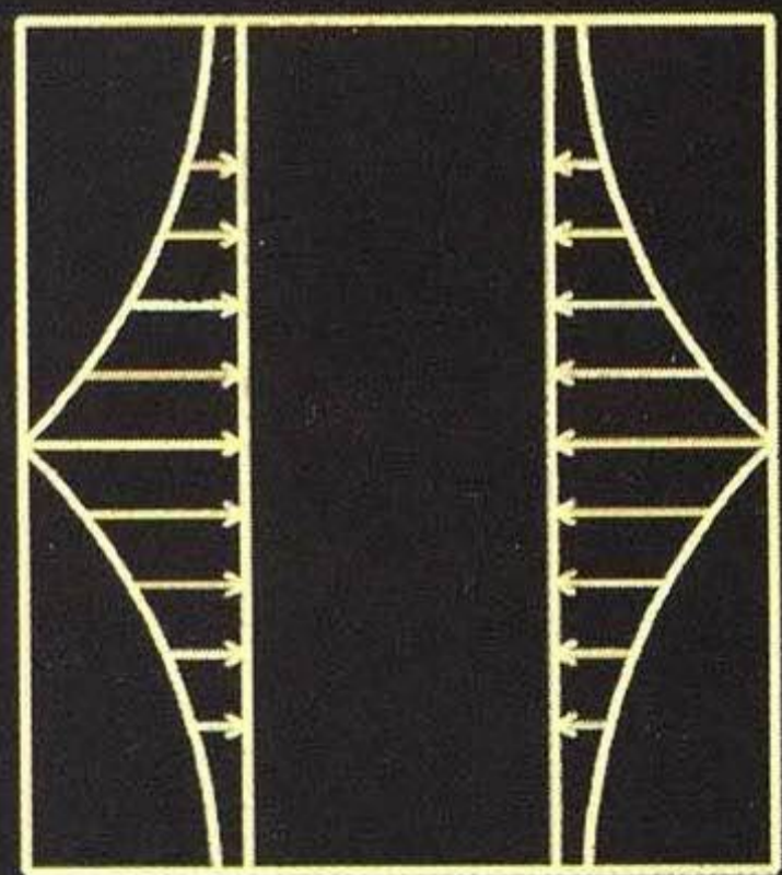
نمودار توزیع تنش فشاری پس از جا زدن در پوسته اول
